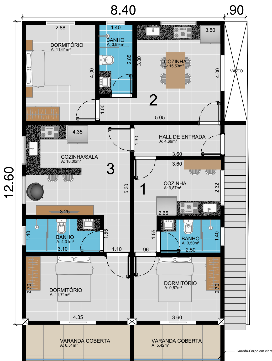
PLANTA PAVIMENTO SUPERIOR esc 1:75
