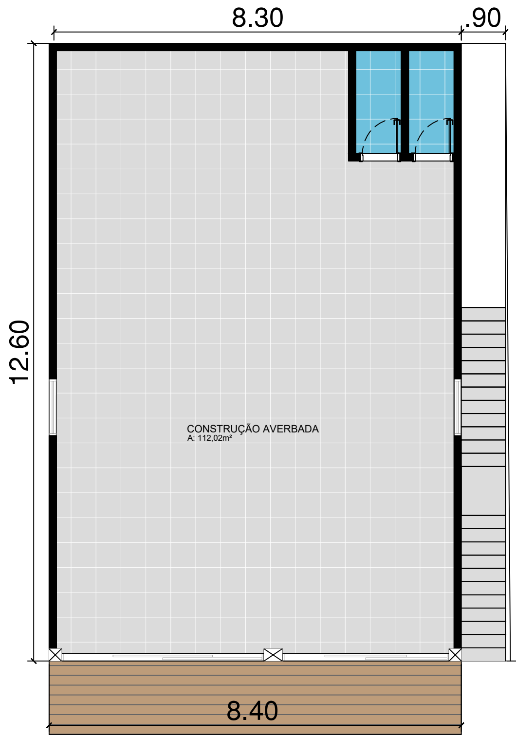
PLANTA PAVIMENTO TÉRREO esc 1:75
